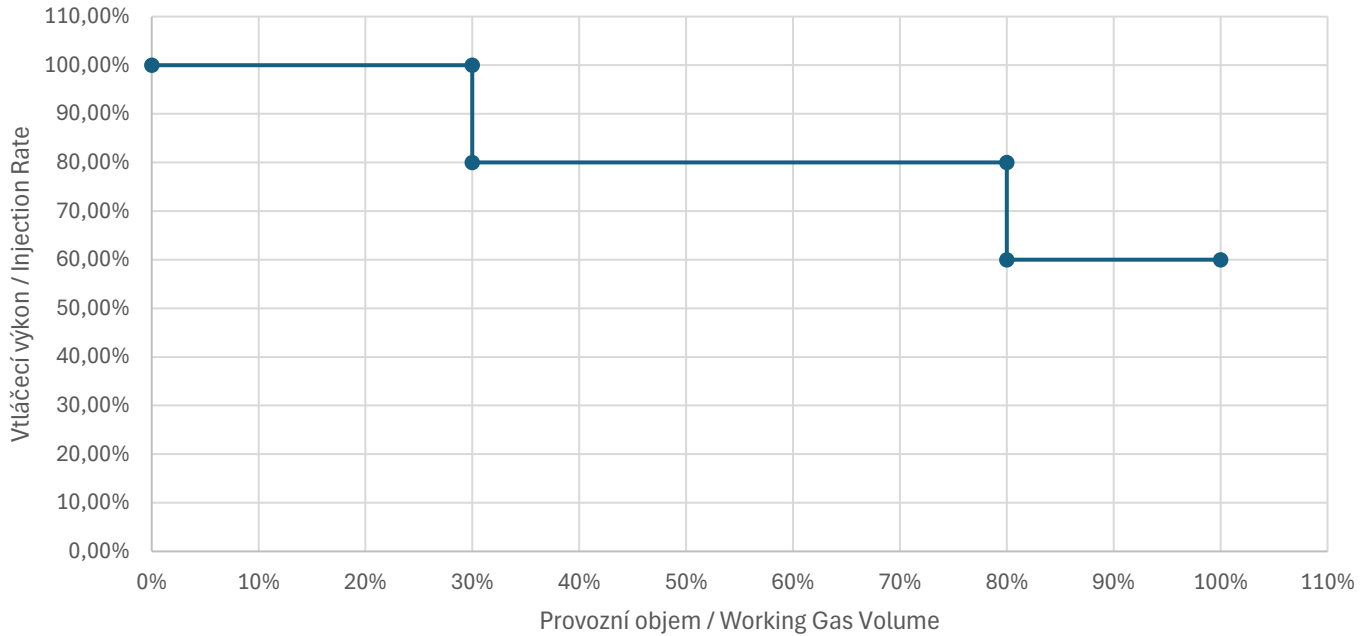
Vtláčeční křivka / Injection Curve
