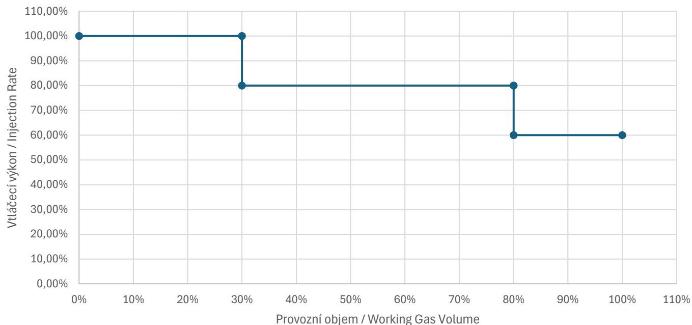
Vtlačecí křivka / Injection Curve
