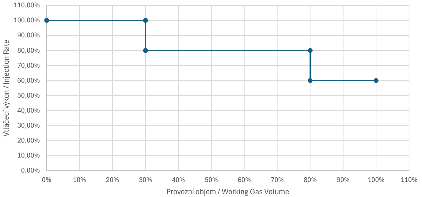
Vtláčečcí křivka / Injection Curve
