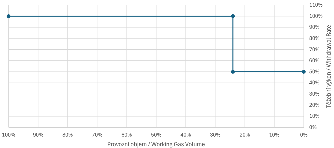
Těžečbní křivka / Withdrawal Curve
