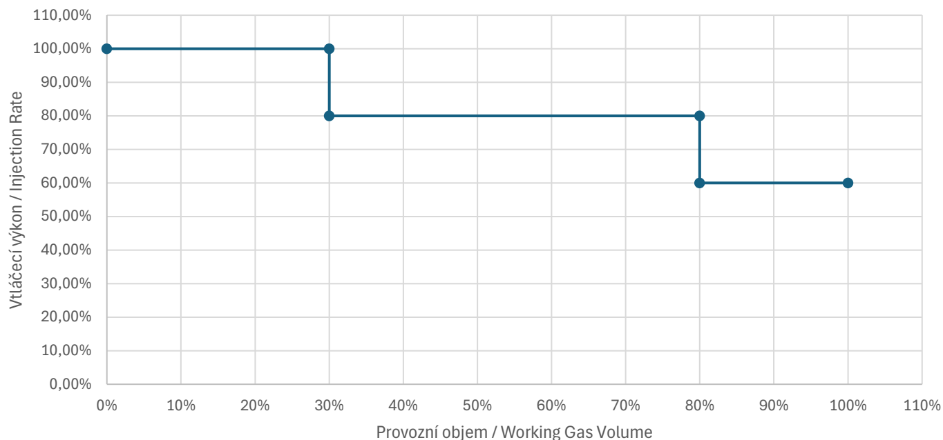
Vtláčeí křívka / Injection Curve
