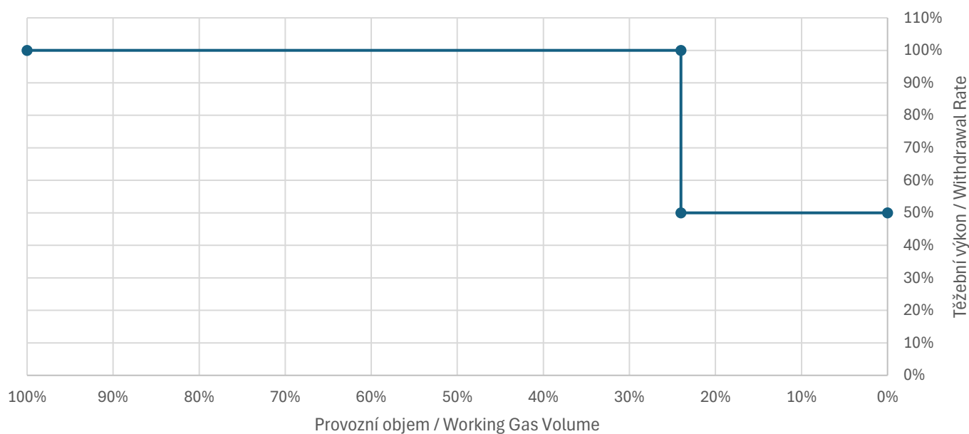
Těžeí křívka / Withdrawal Curve
